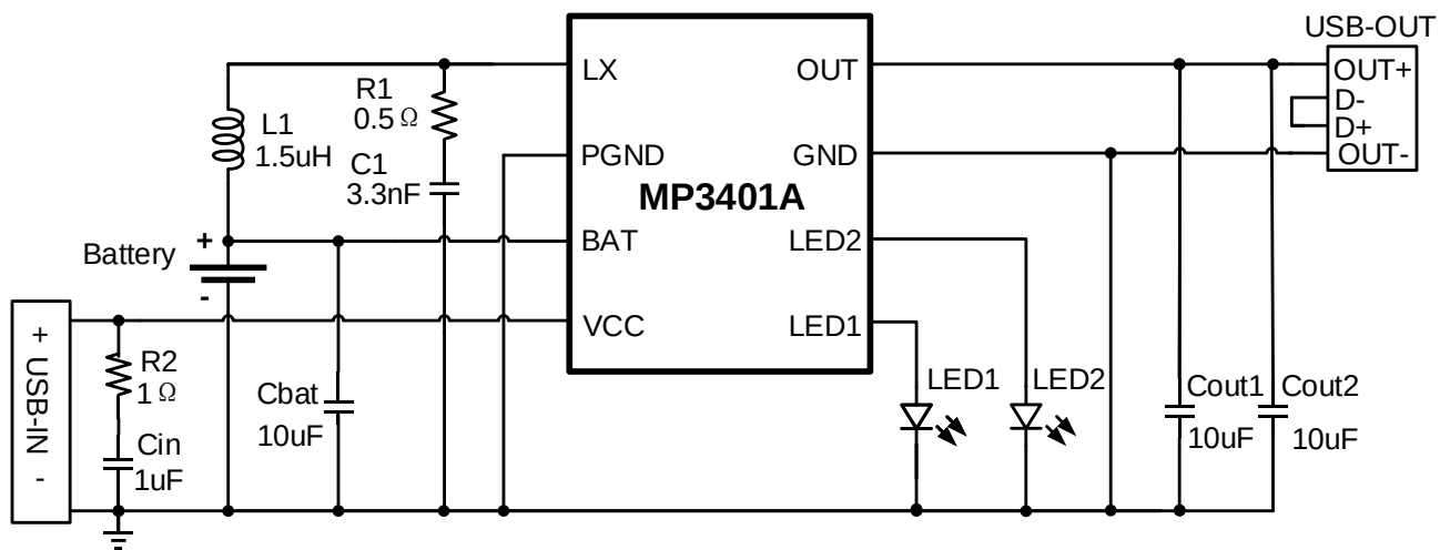
MP3401A 典型应用电路
